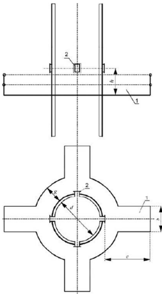
1 - рабочая площадка; 2 - входное отверстие; b - длина рабочей зоны; d - внутренний диаметр газохода; e - ширина рабочей зоны; g - ширина прохода между рабочими зонами; h - минимальная высота свободной зоны над рабочей площадкой
