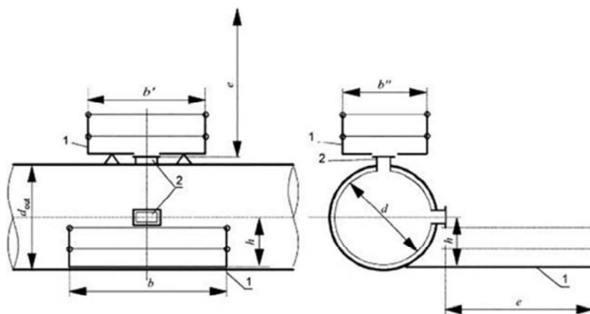
1 - рабочая площадка; 2 - входное отверстие; b , b' , b'' - длина рабочей зоны; d - внутренний диаметр газохода; d_{вн} - наружный диаметр газохода; e - ширина рабочей зоны; h - минимальная высота свободной зоны над рабочей площадкой
