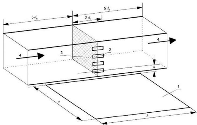
Рисунок Л.5 - Пример рабочей площадки и размещение входных отверстий в вертикальном прямоугольном газоходе
